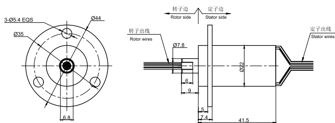
MC330-IP65 图纸
