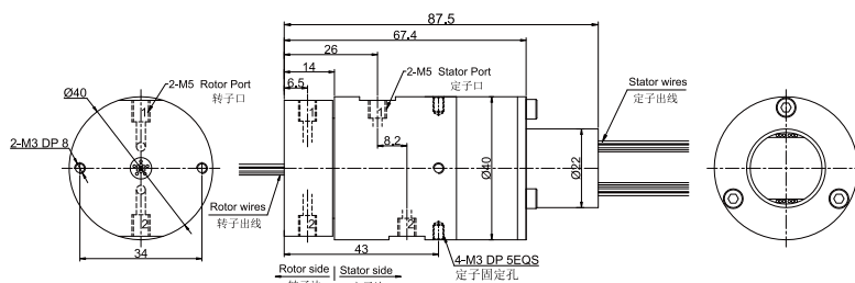
MQR2-S24 尺寸图 2进2出, M5牙 + 24路信号(2A)
